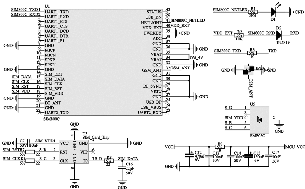
图3 通信模块电路原理图
