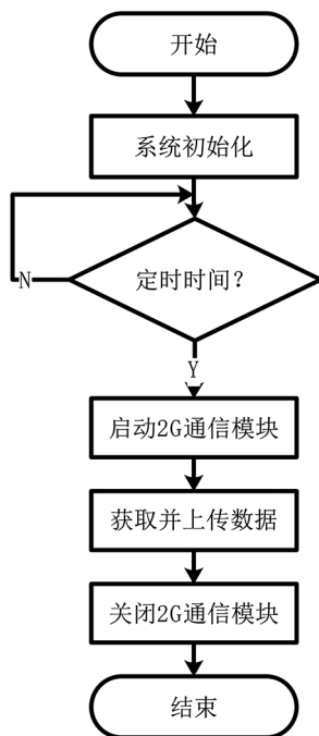
图5 程序设计流程图
