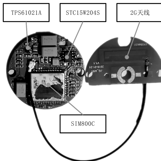
图6 硬件终端电路实物图
