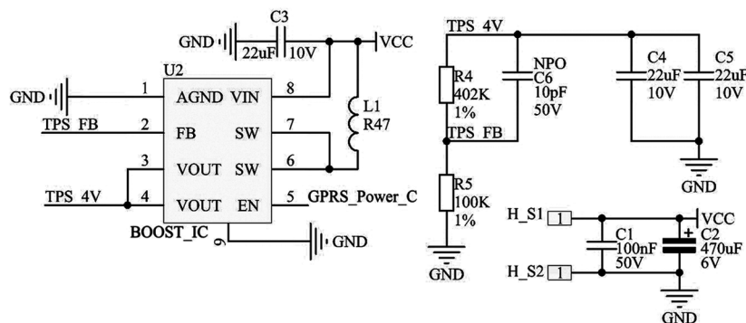
图2 电源模块电路原理图
