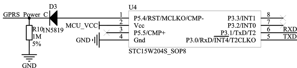
图4 STC15W204S 外围电路原理图
