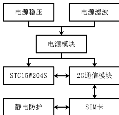
图1 硬件终端系统结构框图
